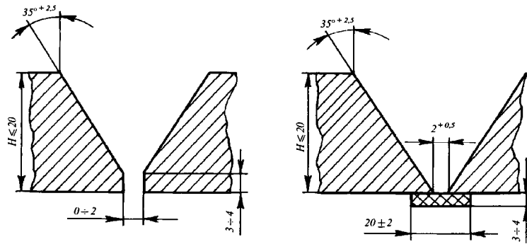
Рис. 11.2.10.8-1 V-образная разделка кромок
