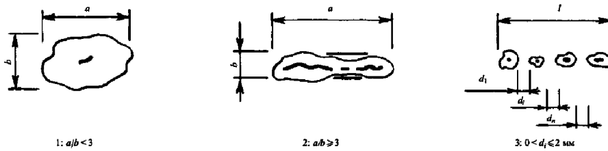
Рис. 11.1.10.4 Тип индикаторного следа: 1 – круглый; 2 – линейный; 3 – рядный
