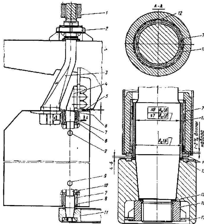
Рис. 6.1.1-3 Рулевое устройство со съемным рудерпостом: 1 — румпель; 2 — подшипник баллера; 3 — баллер; 4, 6 — болты фланцев съемного рудерпоста и пера руля; 5 — ограничитель подъема пера руля; 7 — наборы подшипников пера руля; 8 — отливки пера руля; 9 — крышки для осмотров; 10 — съемный рудерпост; 11 — пятка ахтерштевня; 12 — упорная планка; 13 — облицовка съемного рудерпоста; 14 — упорные кольца; 15 — уплотнения конуса; 16 — гайка съемного рудерпоста; 17 — стопор
