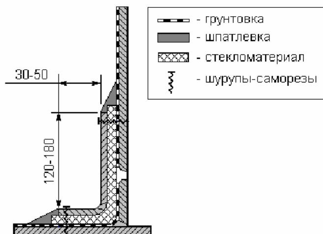
Рис. 8.3.3-1 Металлическая накладка в углах соединения стенок надстройки с палубой
