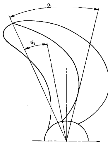
Рис. 11.2.3.3-2 Угол откидки:
