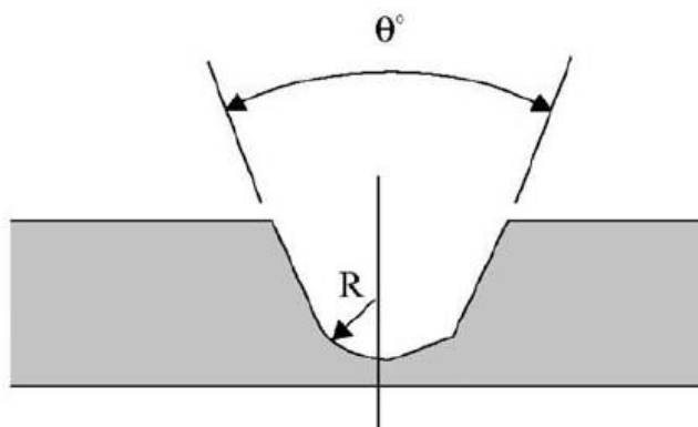
Рис. 2.1.5-4 Подготовка под сварку (слева – разделка U-образной формы, справа – разделка V-образной формы)
