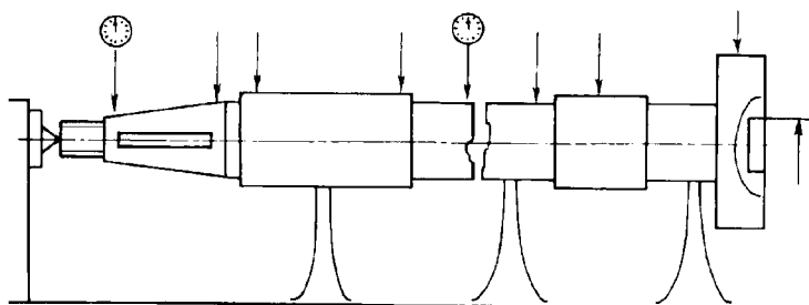
Рис. 10.6.5.1-3 Схема измерения соосности рабочих и нерабочих поверхностей гребного вала при медленном вращении с использованием люнетов токарного станка
