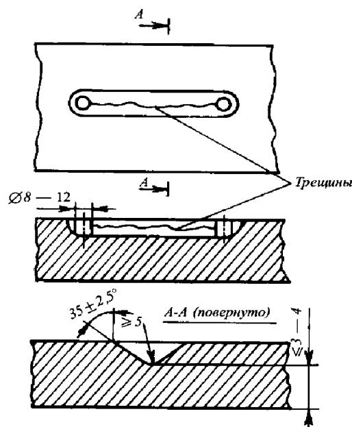
Рис. 11.2.10.5 Подготовка под заварку несквозных трещин
