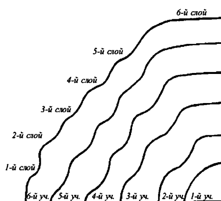
Рис. 11.1.7.34 Валики наплавки
