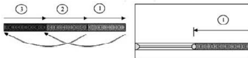
Рис. 2.1.5-3 Последовательность заварки трещин длиной менее 300 мм
