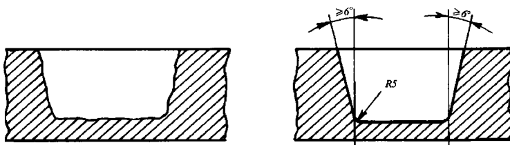
Рис. 11.1.7.16-3 Углы разделки широких раковин
