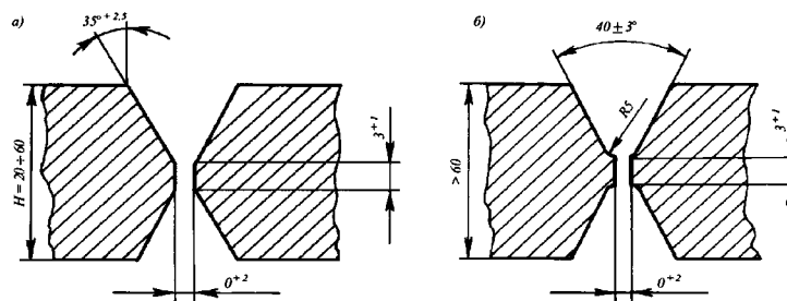
Рис. 11.2.10.8-2 Разделка кромок: а — X-образная; б — Ж-образная
