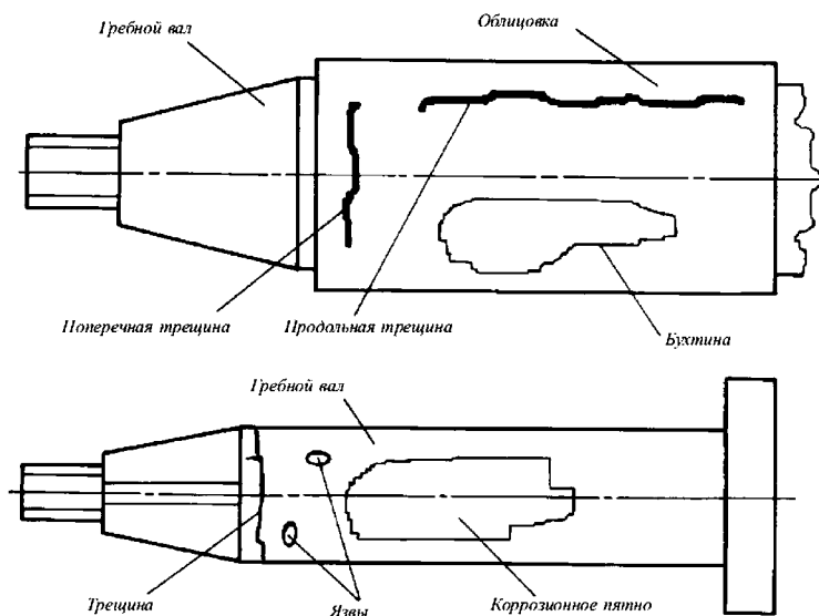
Рис.10.6.1.1 Типовые повреждения гребных валов
