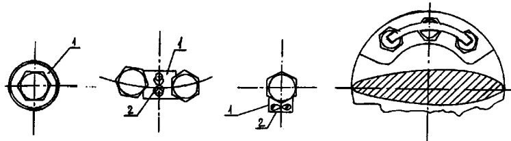
Рис. 11.2.12.8 Варианты стопорения гаек для шпилек съемных лопастей: 1 — стопорная планка; 2 — проволочный шплинт
