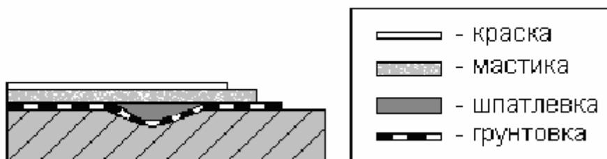
Рис. 8.4.2 Эпоксидное мастичное покрытие
