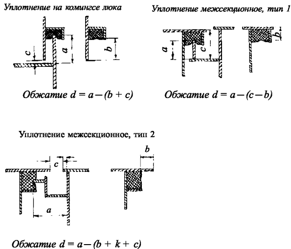
Рис. 5.3.3 Определение величины обжатия резинового уплотнения
