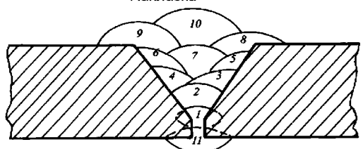
V-образная разделка
