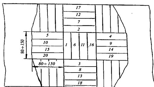
Рис. 11.2.10.16-1 Очередность наложения сварных швов при наплавке
