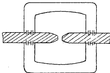
Рис. 11.1.7.20-1 Гребенки для устранения угловых деформаций
