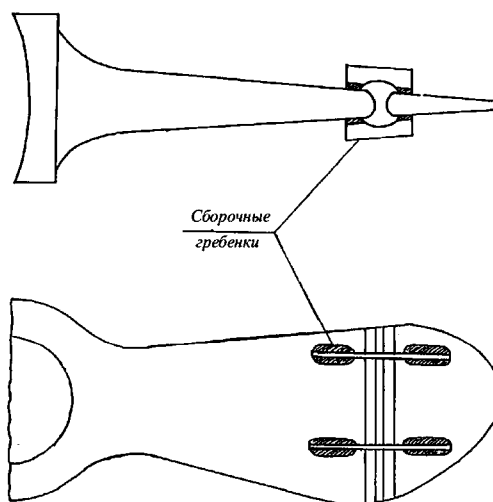
Рис. 11.2.10.17 Установка сборочных гребенок для приварки лопастных наделок
