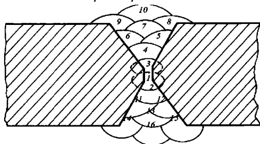
X-образная разделка
