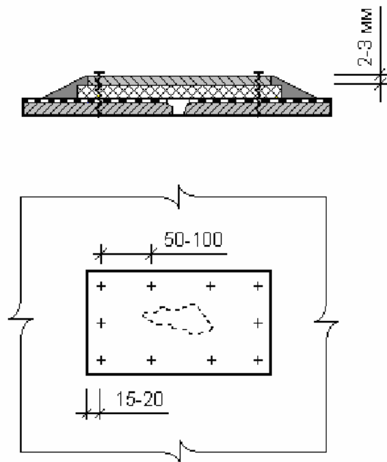
Рис. 8.3.3-2 Металлическая накладка на плоских участках надстройки
