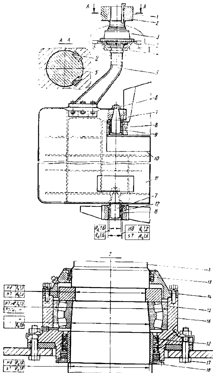
Рис. 6.1.1-7 Руль навесного типа:
