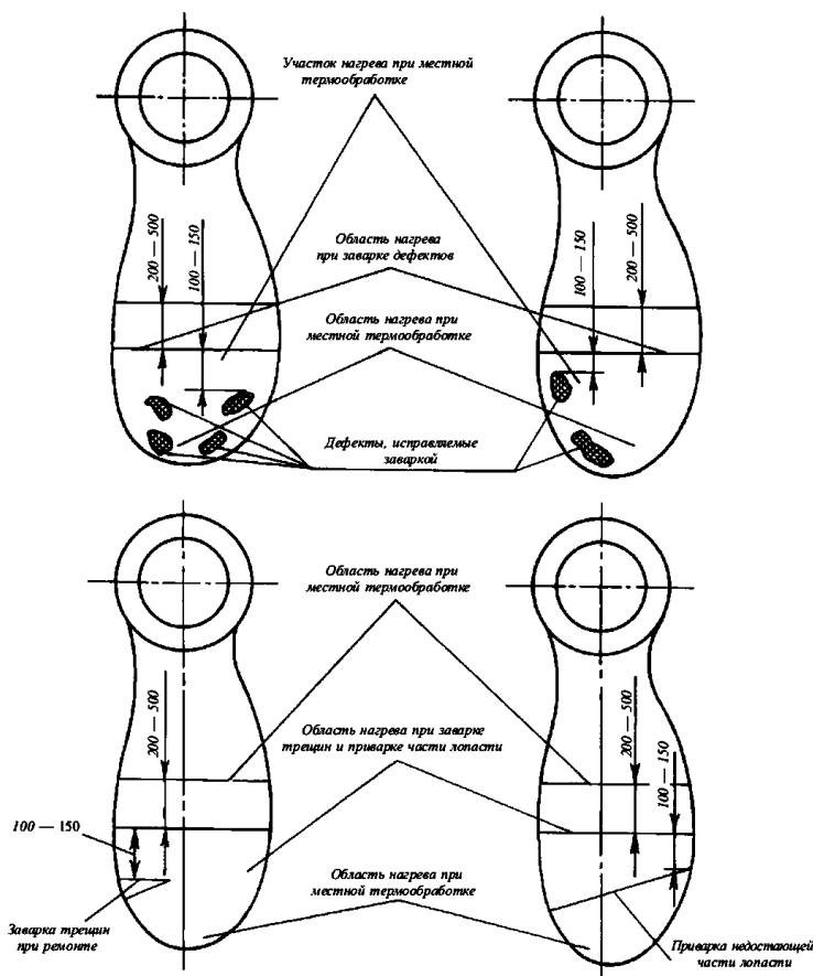
Рис. 11.2.11.7 Участки нагрева при местной термической обработке
