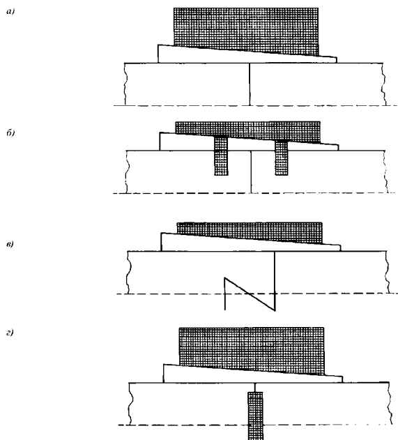
Рис. 10.8.3.1 Некоторые типы бесфланцевых соединений валов:
