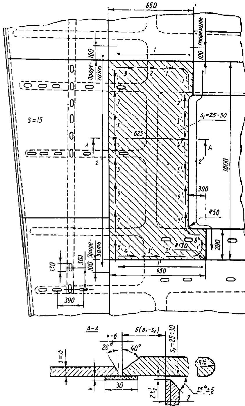
Рис. 6.4.1-2 Установка усиленного листа обшивки пера руля
