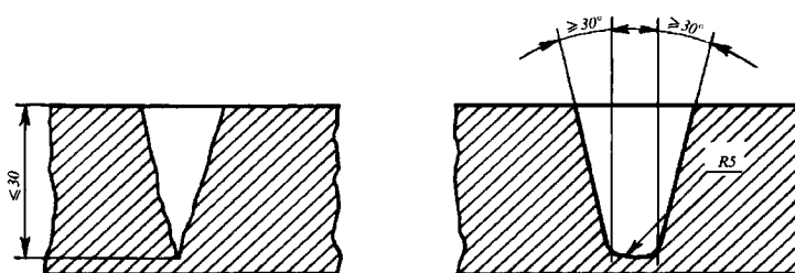
Рис. 11.1.7.15-1 Разделка несквозных трещин при глубине дефекта до 30 мм включительно
