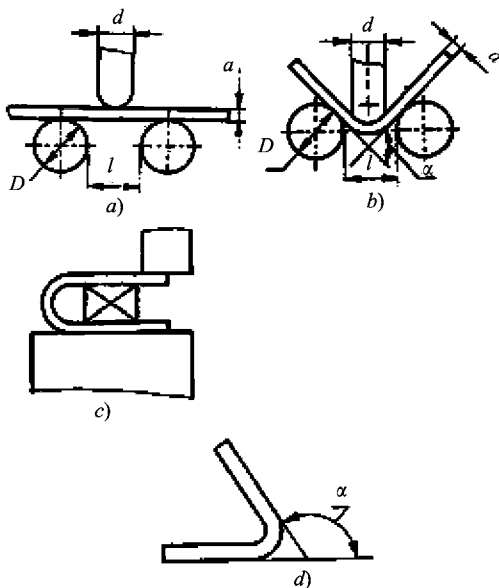
Fig. 3 Bend test
