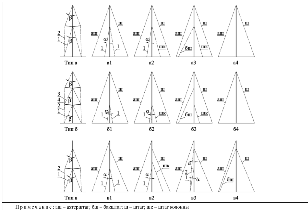
Типы такелажа
