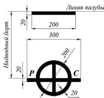
Рис. 6.2.2.1 Грузовая марка
