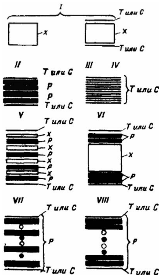
Рис. 6.1.1 Схемы армирования
