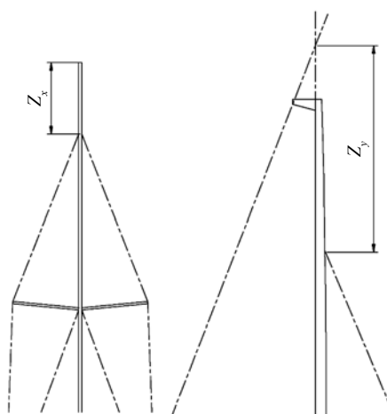
Рис. 5.4.1.6 Размеры топа мачты
