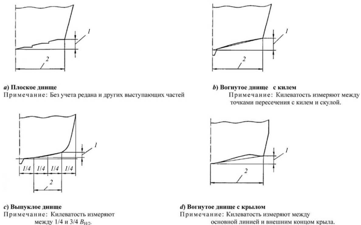
Рис. 3.2.21 Определение килеватости Обозначения: l – высота; 2 – ширина. Вычисление угла килеватости: \beta = \arctg (l:2)
