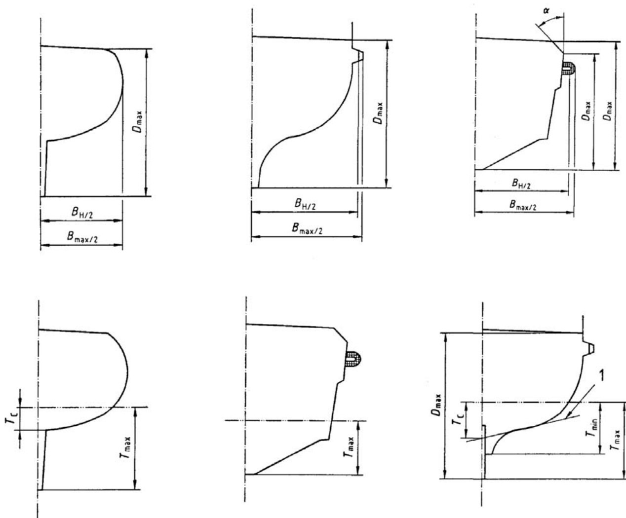
Рис. 3.2.7 Определение размерений B_{max} , B_{пр} , D и T ( d )
