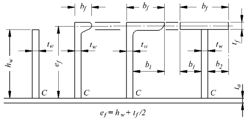
Fig. 7.10.6.31 Dimensions of stiffener
