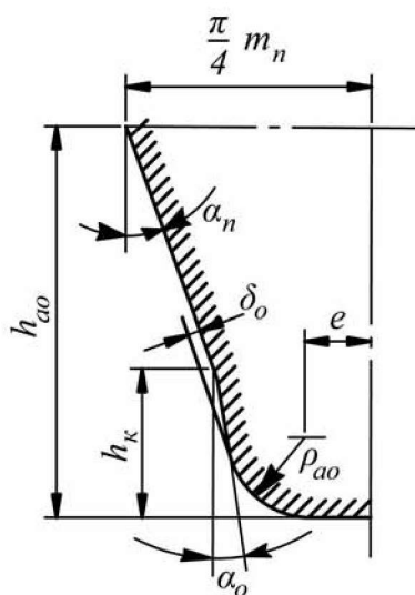
Fig. 4.2.2.7.3.2-3 Protuberance hob
