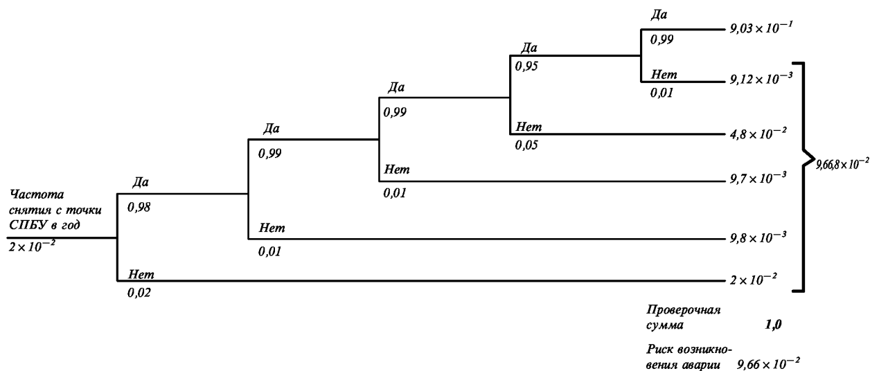
Дерево событий при транспортировках СПБУ и ППБУ
