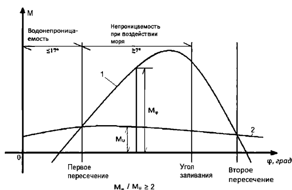
Рис. 2.6.2.1.4 Кривые восстанавливающего момента (1) и ветрового кренящего момента (2)
