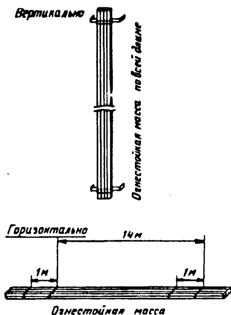
Рис. 16.8.4.3.2-1 Защита кабельной трассы огнестойкой массой
