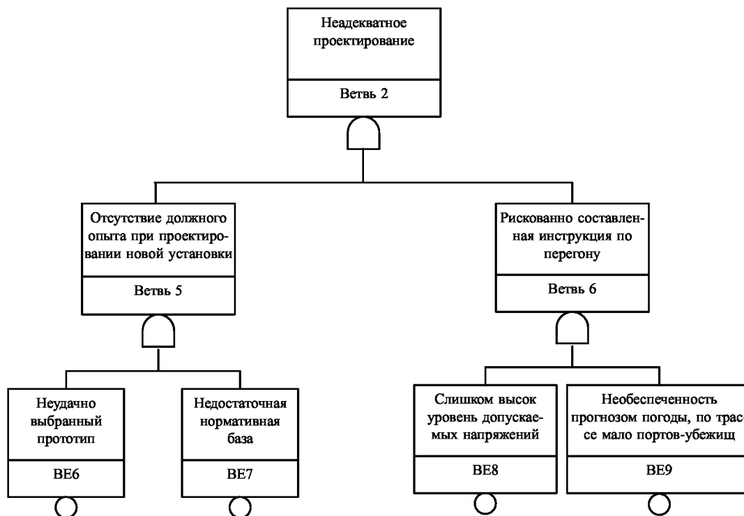
Продолжение построения дерева ошибок и неполадок
