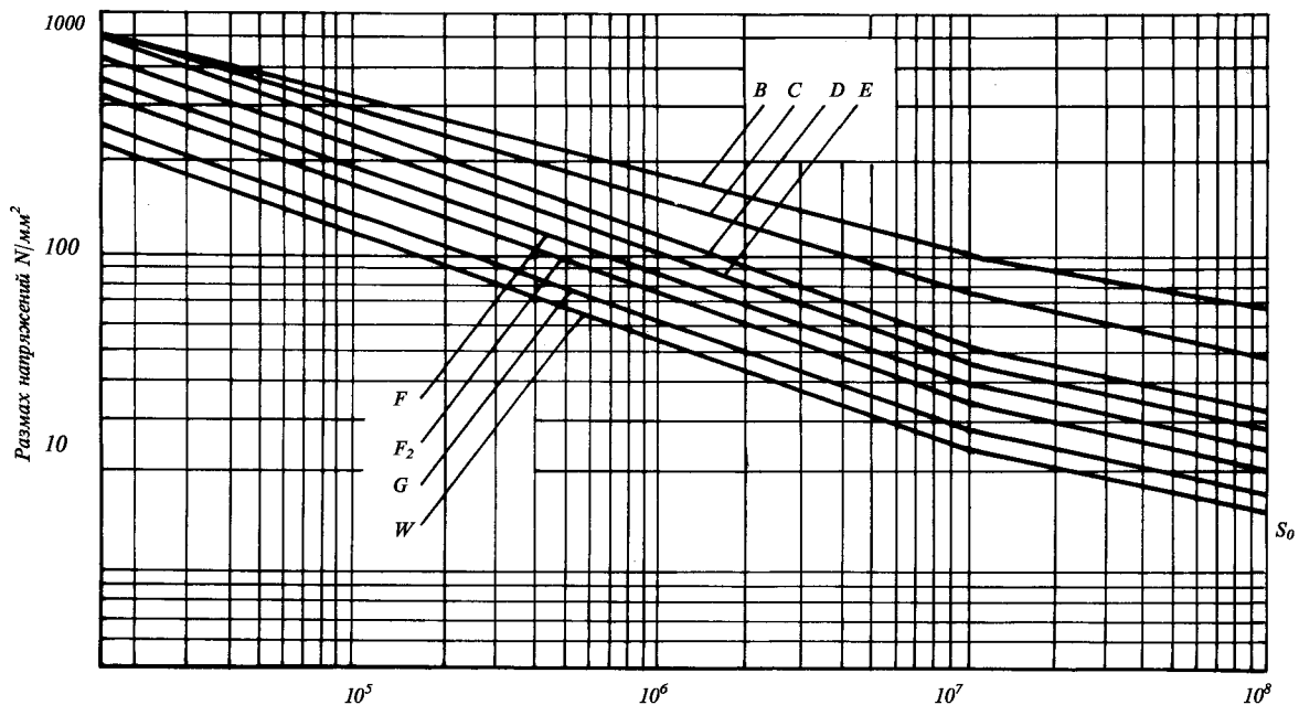
Рис. 2.4.4.8-1 Кривые усталости
