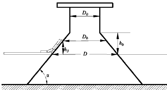
Рис. 3.3.2.3.18-1 Платформа с расширяющимися вниз коническими бортами
