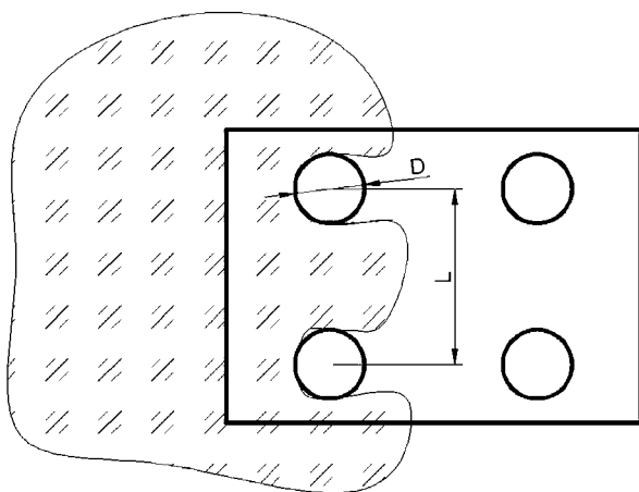
Рис. 3.3.2.3.11 Многоопорная платформа
