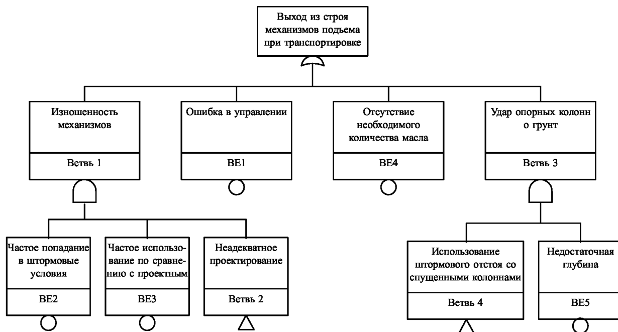
Начальное построение дерева ошибок и неполадок
