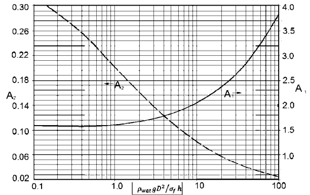
Рис. 3.3.2.3.18-2 Значения коэффициентов A_1, A_2
