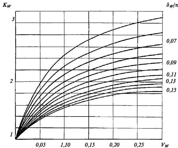
Рис. 3.1.3.2 Коэффициент динамичности ветровых нагрузок
