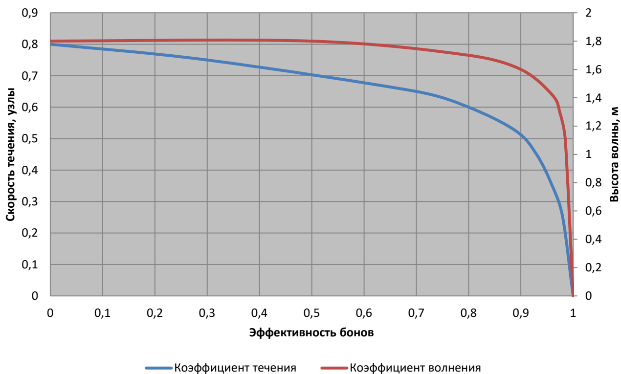
Рисунок 3Б – Характеристики эффективности цилиндрических БЗ категории I – III
