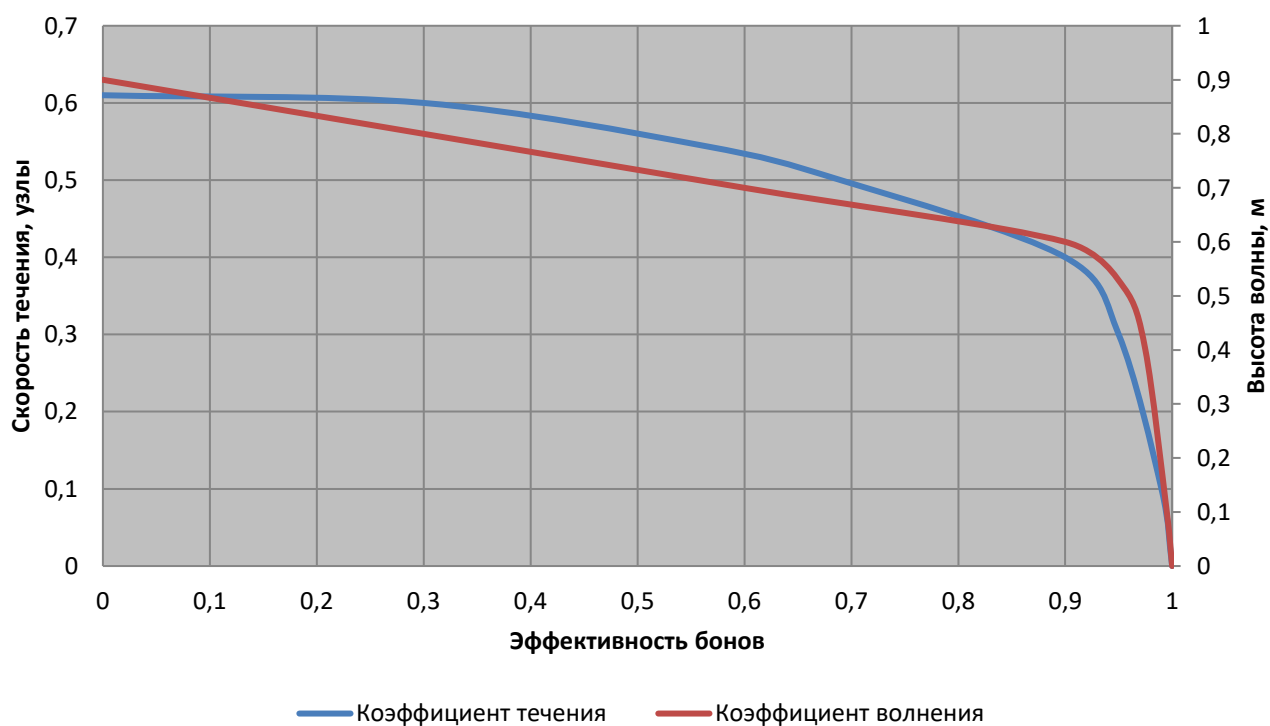
Рисунок 4Б – Характеристики эффективности БЗ постоянной плавучести категории I - III
