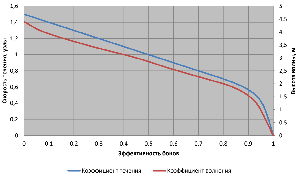
Рисунок 1Б – Характеристики эффективности цилиндрических БЗ категории IV – V
