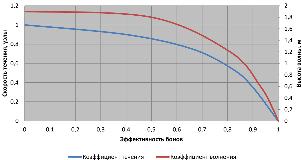
Рисунок 2Б – Характеристики эффективности БЗ постоянной плавучести категории IV - V
