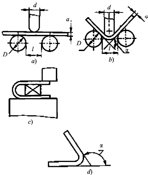
Fig. 3 Bend test
