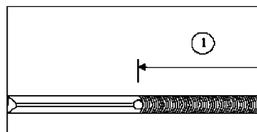
Рис. 6.8в Последовательность заварки трещин длиной менее 300 мм
