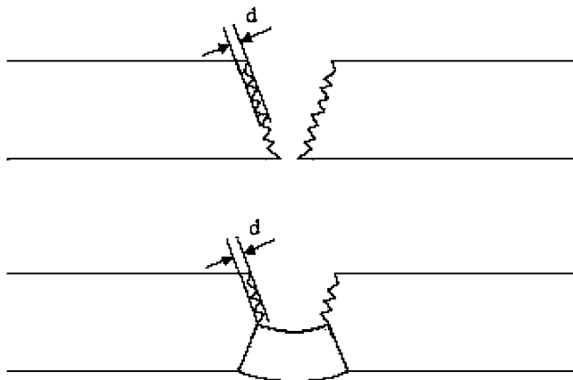
Рис. 6.1 Шероховатость кромок
