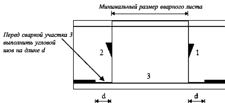
Рис. 6.4 Последовательность приварки вварных листов на ребра жесткости
