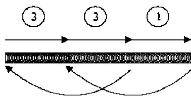
Рис. 6.8а Обратнo-ступенчатая сварка
