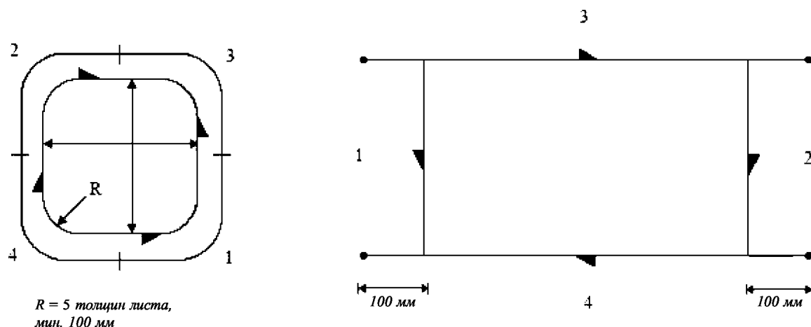
Рис. 6.2 Последовательность сварки в случае применения сварных листов
