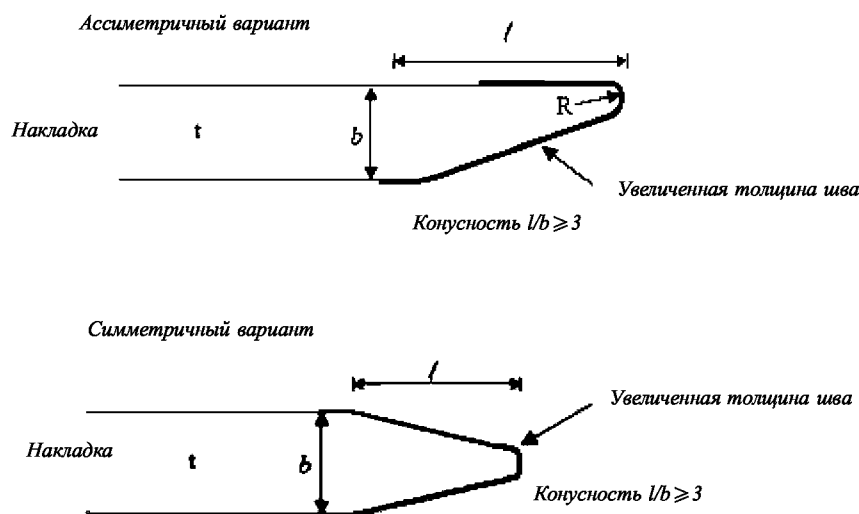
Рис. 6.6 Применение накладок
