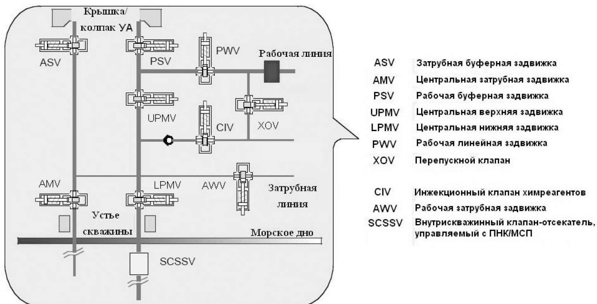
Рис. 1 Типовой комплект оборудования и арматуры
