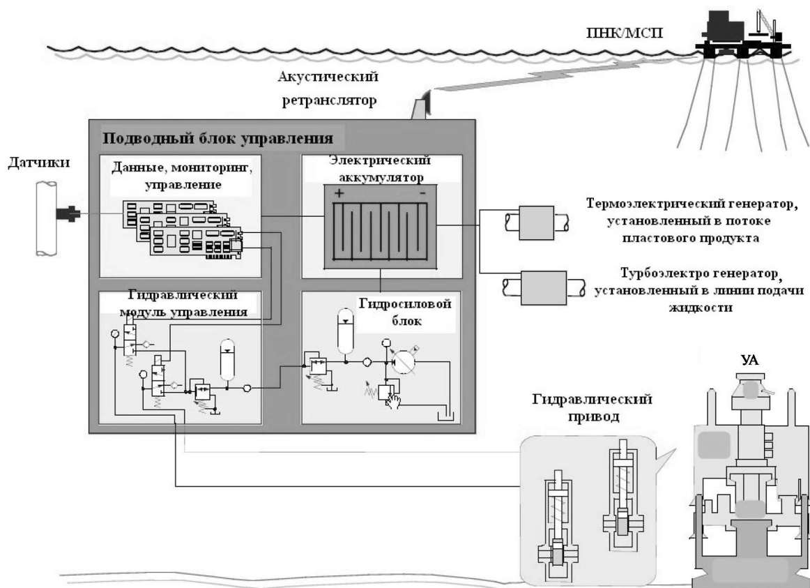
Рис. 7 Автономные системы (SPARCS)
