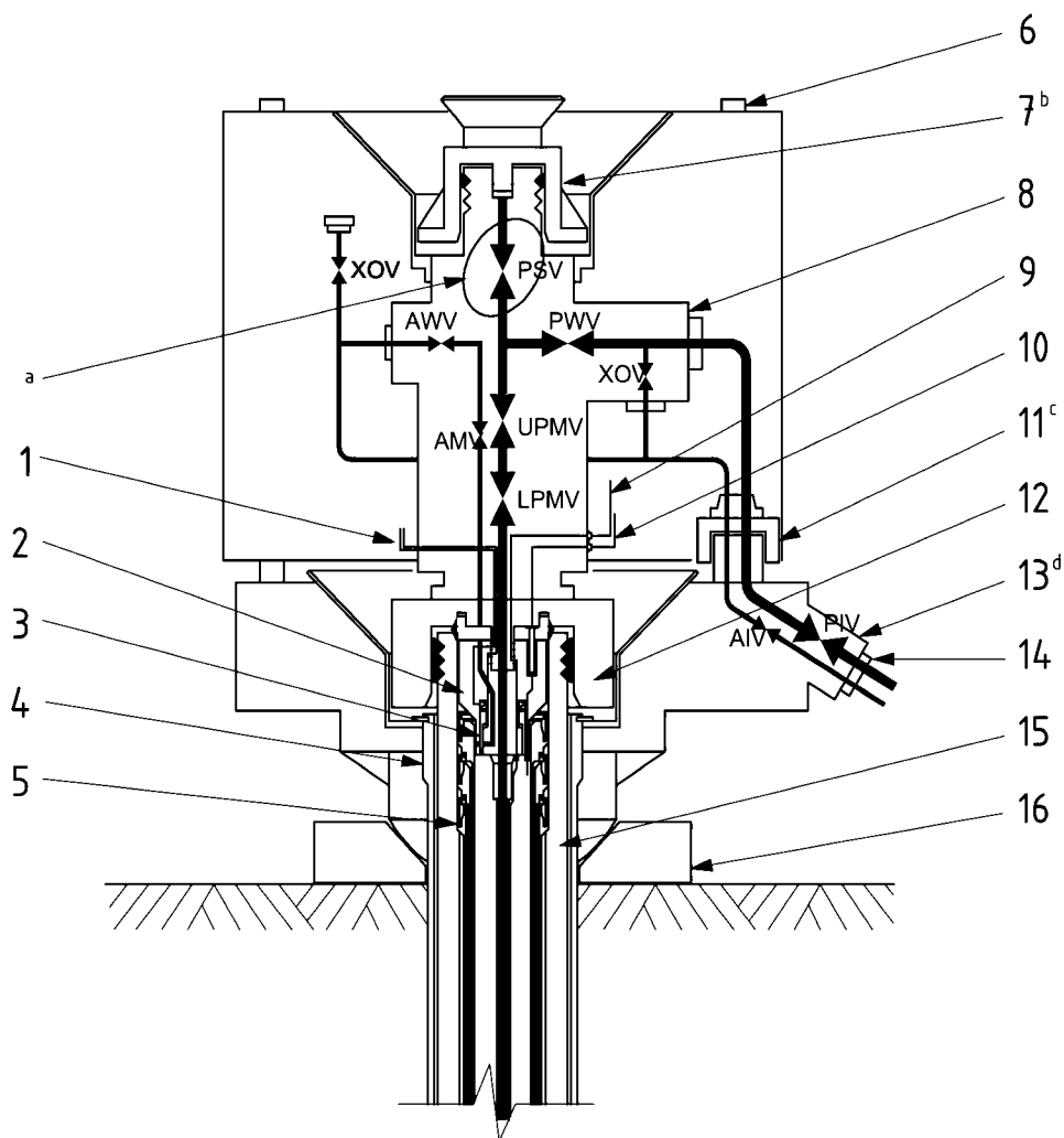
Рис. 3 Вертикальная устьевая арматура (VXT) концентрического типа
