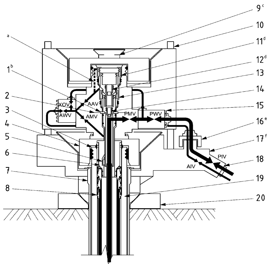
Рис. 5 Горизонтальная устьевая арматура (НХТ)
