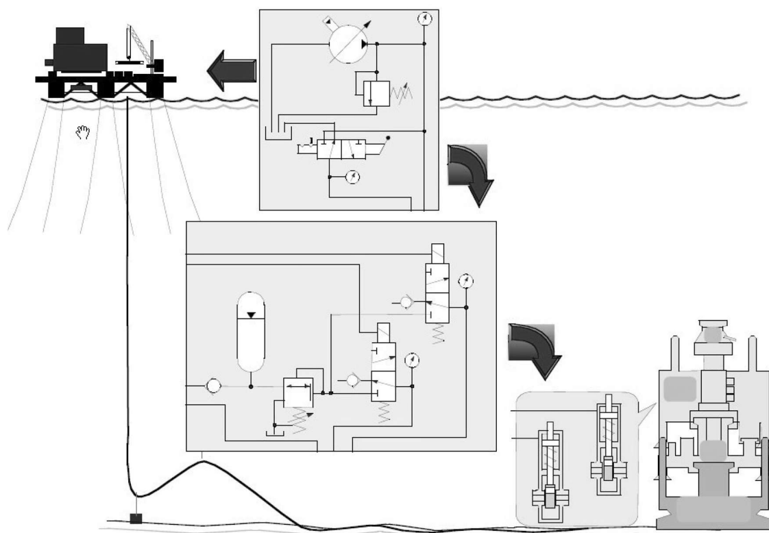
Рис. 5 Электрогидравлические системы с непосредственным приводом
