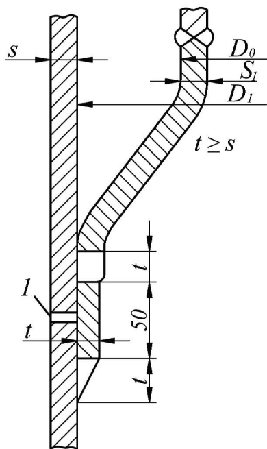
Рис. 2.2.2.8: l — не менее четырех отверстий \varnothing 10 , равномерно распределенных по обечайке
