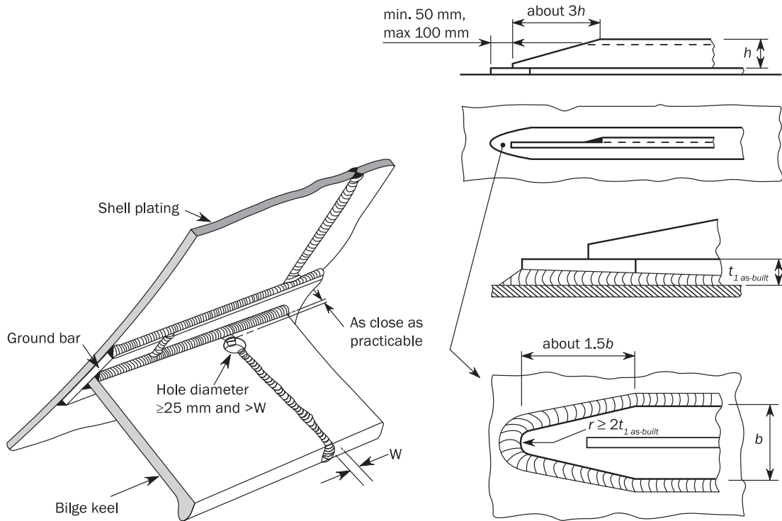
Figure 10 : Bilge keel
